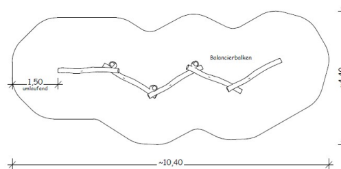
Draufsicht
